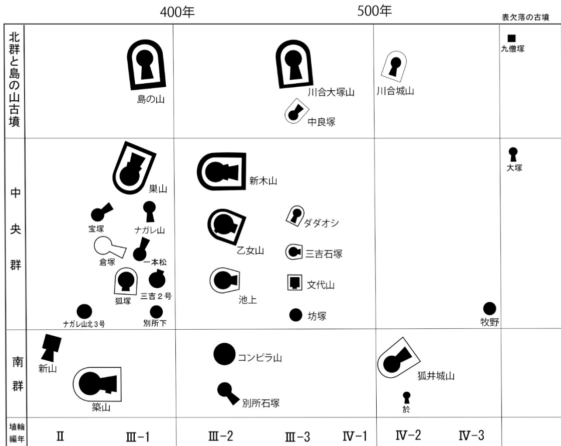
図 2-17 馬見古墳群の編年図
