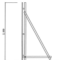
敷地外周仮囲い フラットパネルH=2000
