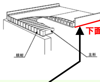
主桁の損傷（ひびわれ）
