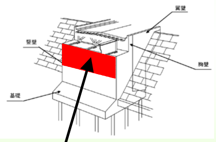
橋台の損傷（ひびわれ）
