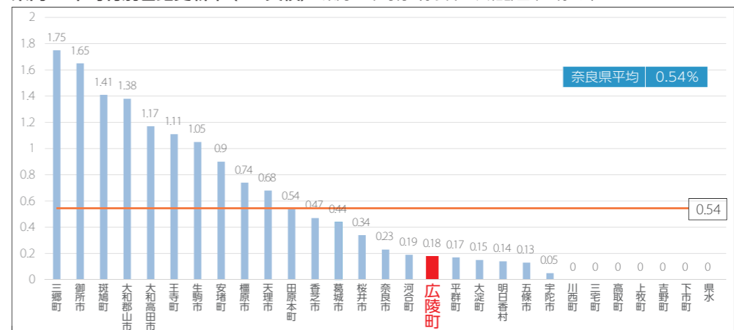
県内26市町村別管路更新率 (R2実績) ※県内26市町村 (奈良市、大和郡山市を除く。)
