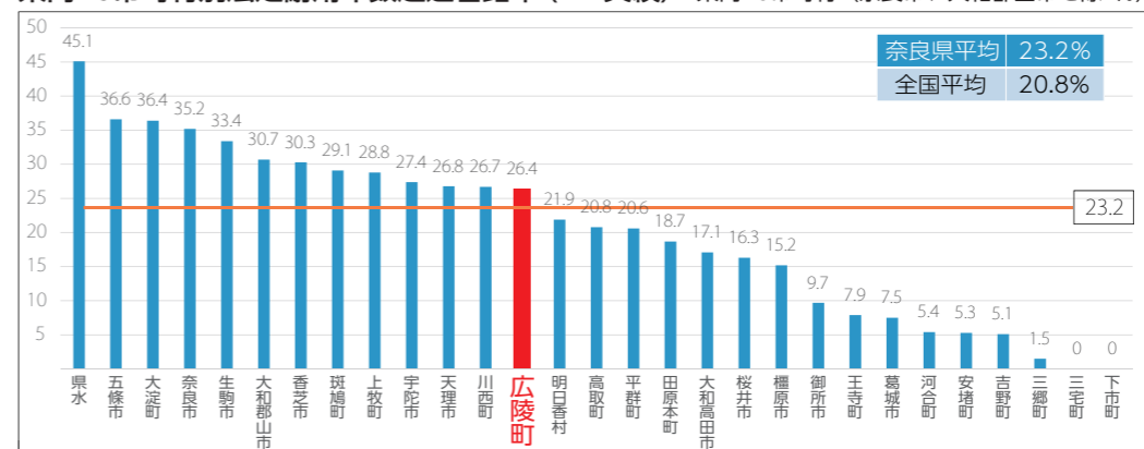
県内26市町村別法定耐用年数超過管路率 (R2実績) ※県内26市町村 (奈良市、大和郡山市を除く。)
